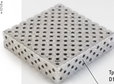
Плита стола с системными отверстиями D16 по двойной координатной сетке 50 x 50 мм
