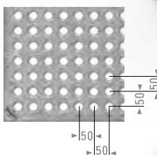
Плита стола с системными отверстиями D22, расположенными по координатной сетке 50 × 50 мм
