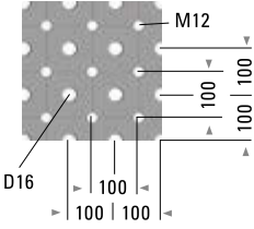
Опция: сварочный стол с диагональной координатной сеткой 50 x 50 мм и резьбой M12
